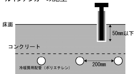
ホールインアンカーの施工
